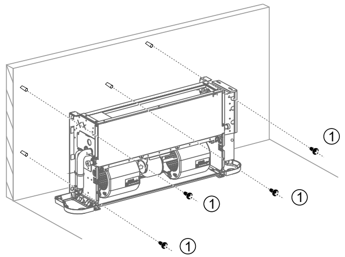
Fijación del cuerpo de la unidad
