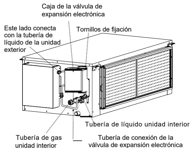
Figura 5.7 Unidad de conductos de alta presión 10.0kW ~15.0kW y procesador de aire fresco 14.0kW
