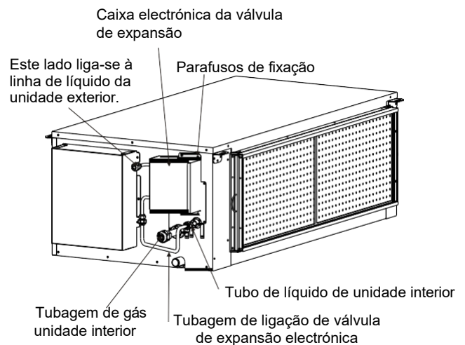
Figura 5.7 Unidade de condutas de alta pressão 10.0kW ~ 15.0kW e processador de ar fresco 14.0kW
