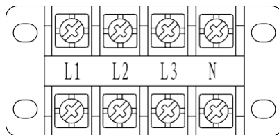
Courant triphasé
