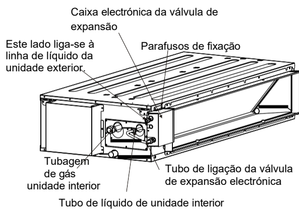
Figura 5.6 Pressão estática padrão e unidade de condutas de alta pressão 7.1kW~9.0kW
