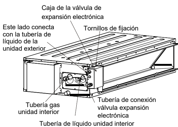
Figura 5.6 Unidad de conductos de presión estática estándar y alta presión 7.1kW~9.0kW
