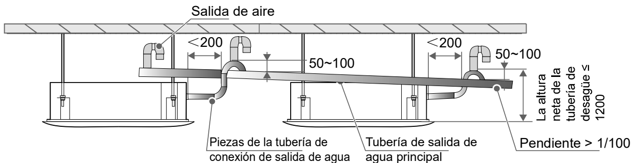
Las tuberías de desagüe de varias unidades se conectan a la tubería de desagüe principal para, a su vez, descargarse a través de la canalización de aguas residuales.
