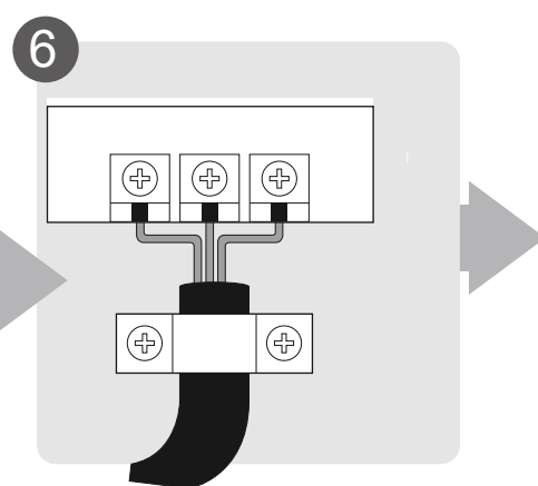
6 Conecte el cableado (no aplicable para algunas ubicaciones en los EE.UU.)
