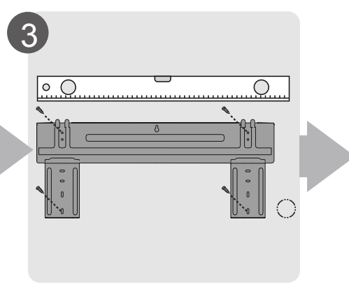
Monte a Placa de Montagem
