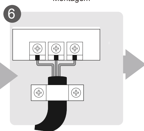
Conecte a Fiação (não aplicável a algumas partes da América do Norte)
