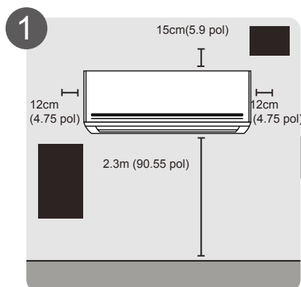
Selecione o Local da Instalação
